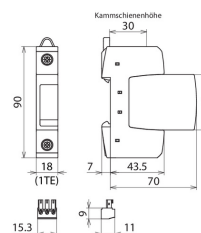
Maßbild DG S ACI 275 FM
