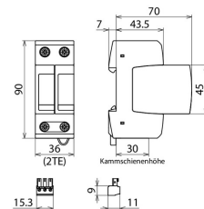
Maßbild DG M TT 2P ACI 275 FM
