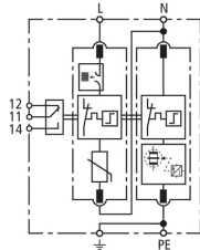
Prinzip Schaltbild DG M TT 2P ACI 275 FM
