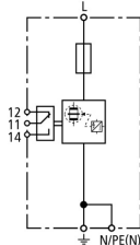
Prinzipialschaltbild DBM 1 CI 440 FM
