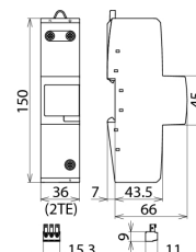
Maßbild DGPM 1 255 FM
